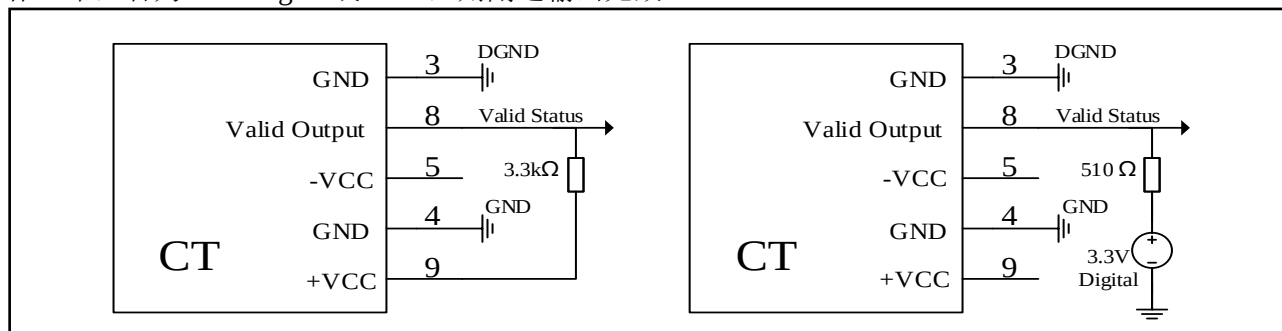
输出状态端口连接图
